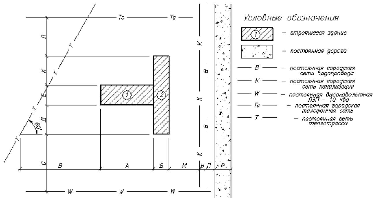
Рис. 5. Схема генплана «В»
