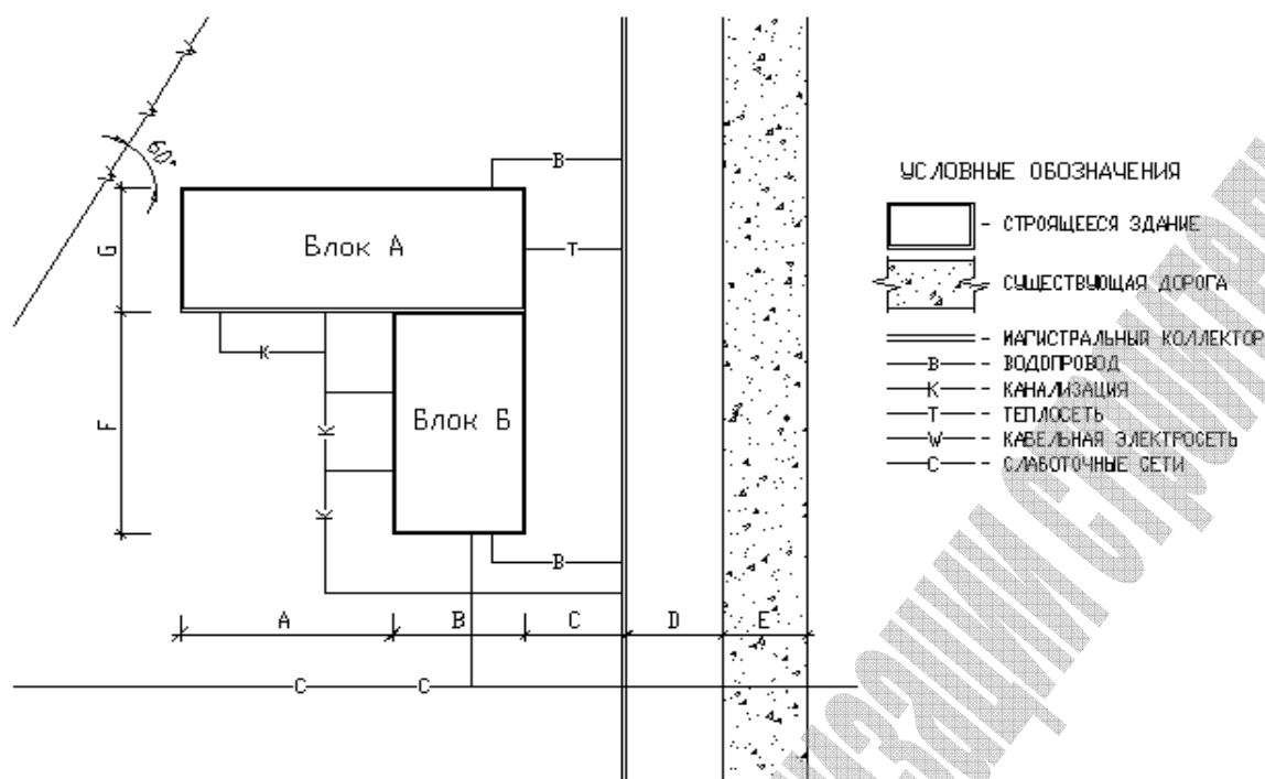
Рис. 3. Схема генплана «А»
