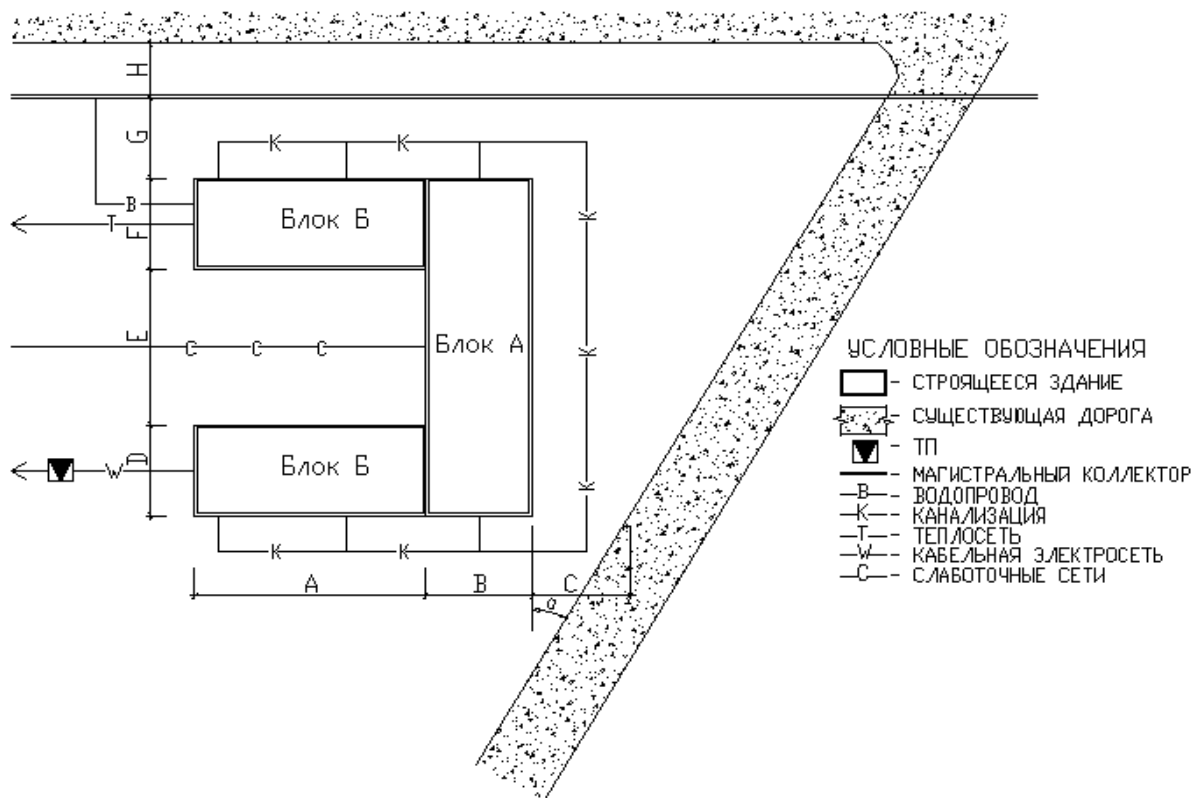
Рис. 4. Схема генплана «Б»
